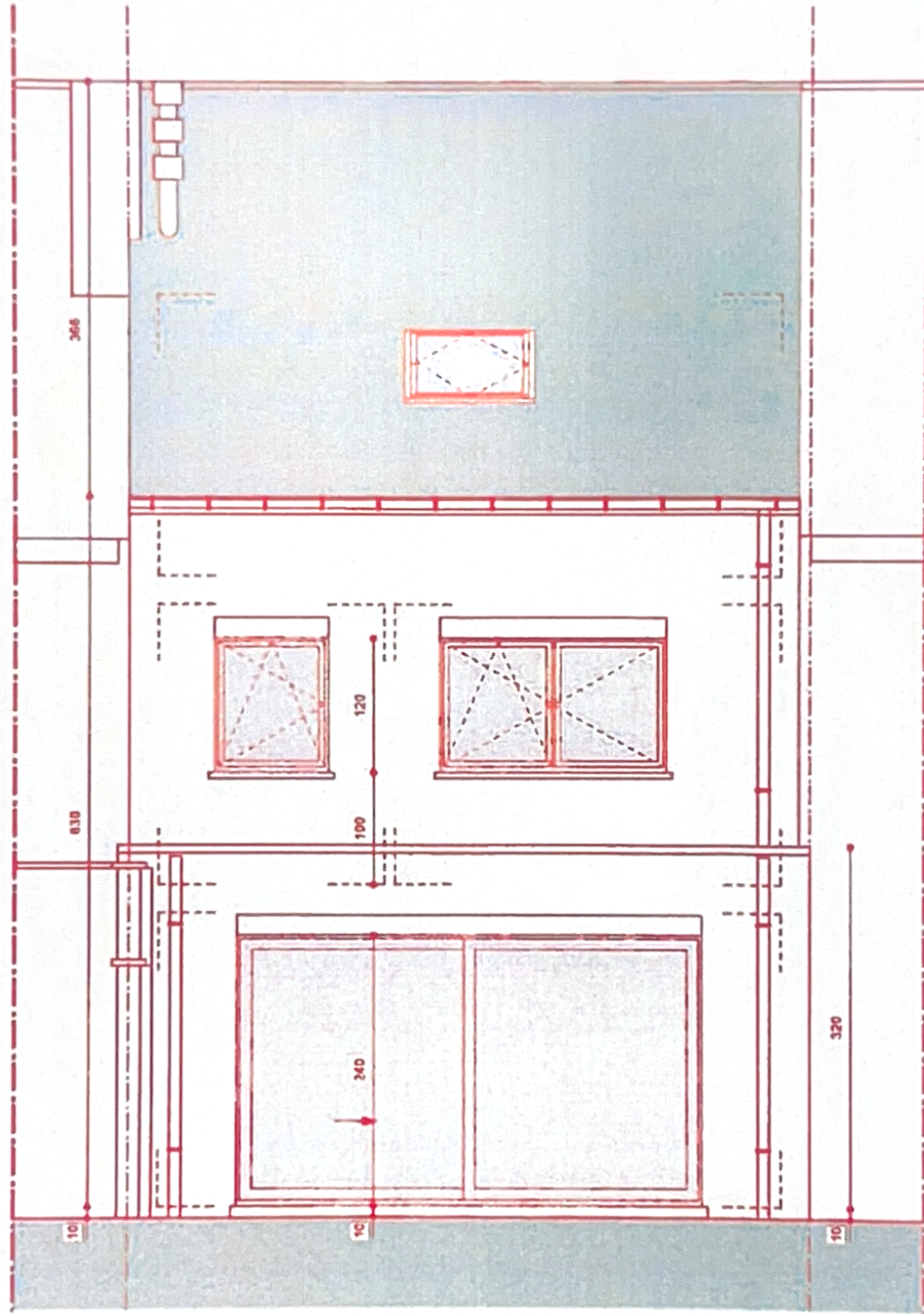
ACHTERGEVEL
