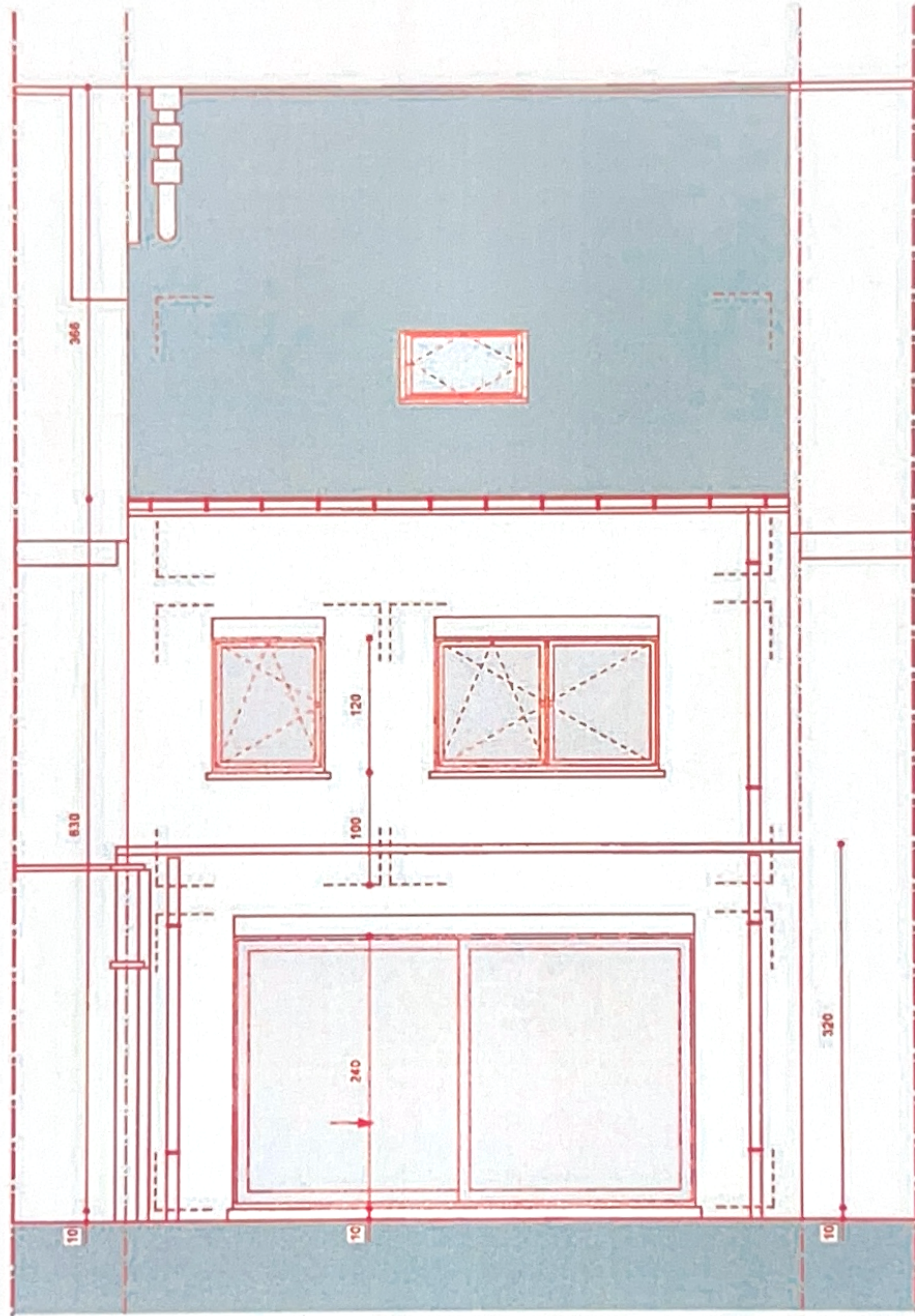
ACHTERGEVEL
